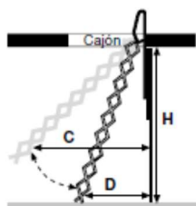
ZX TECHO- Metálica Galvanizada Metálica Galvanizada
