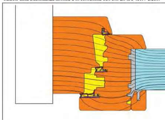
Calcolo della trasmittanza termica U in conformità con UNI EN ISO 10077-2:2007
