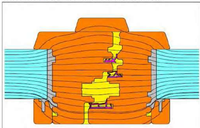
Calcolo della trasmittanza termica U in conformità con UNI EN ISO 10077-2:2007
